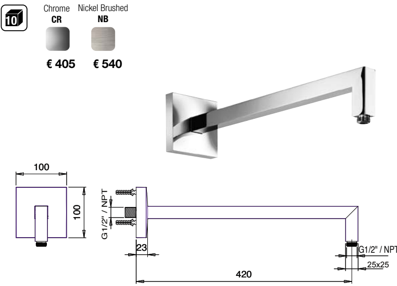
E021053 EMOTION QUADRO RINFORZATO L420 - OTTONE REINFORCED SQUARE EMOTION L420 - BRASS
