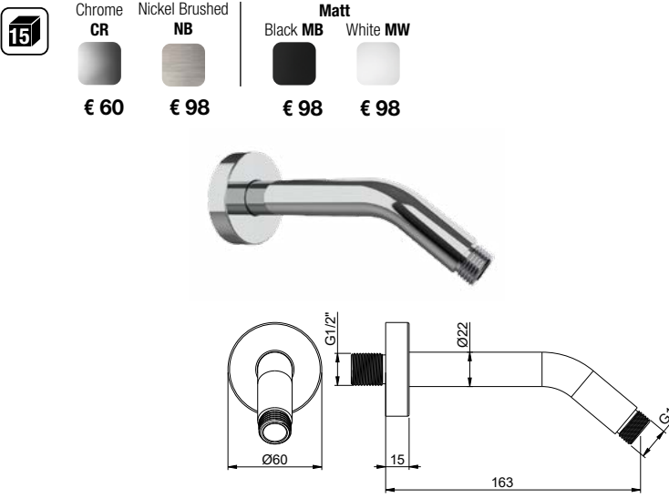
E021058 BRACCIO CORTO CON ROSONE TONDO - OTTONE SHORT ARM WITH ROUND ROSETTE - BRASS
