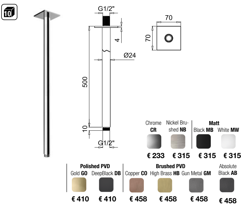
E021110 BRACCIO CON CANNA TONDA E ROSONE QUADRO L 500 - OTTONE ROUND ARM WITH SQUARE ROSETTE L500 - BRASS
