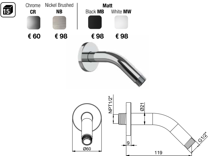
E021105 BRACCIO CORTO CON ROSONE TONDO ATTACCO NPT 1/2" - OTTONE SHORT ARM WITH ROUND ROSETTE NPT 1/2" CONNECTION - BRASS
