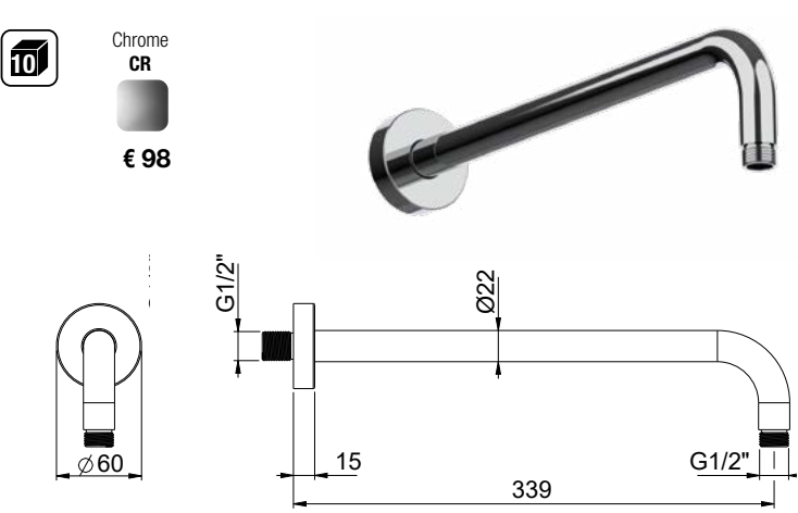
E021118 BRACCIO CON CANNA TONDA E ROSONE TONDO L340 - OTTONE ROUND ARM WITH ROUND ROSETTE L340 - BRASS
