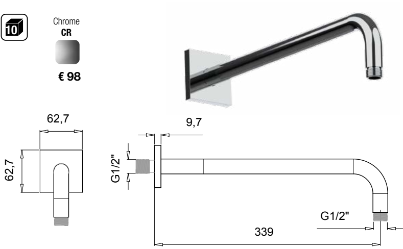
E021124 BRACCIO CON CANNA TONDA E ROSONE QUADRO L340 - OTTONE ROUND ARM WITH SQUARE ROSETTE L340 - BRASS
