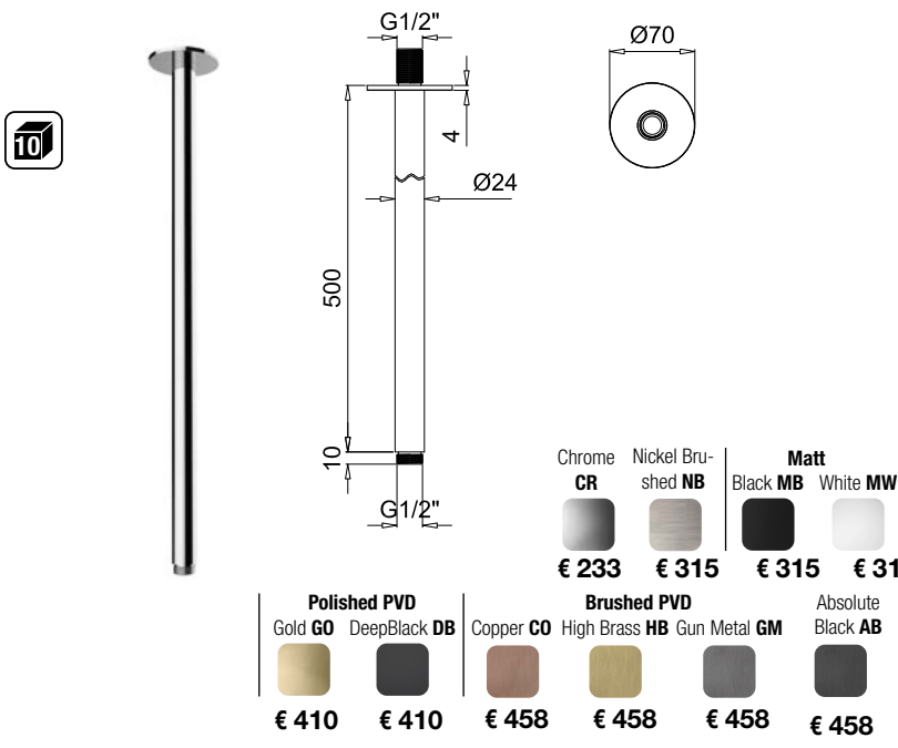
E021111 BRACCIO CON CANNA TONDA E ROSONE TONDO L 500 - OTTONE ROUND ARM WITH ROUND ROSETTE L500 - BRASS
