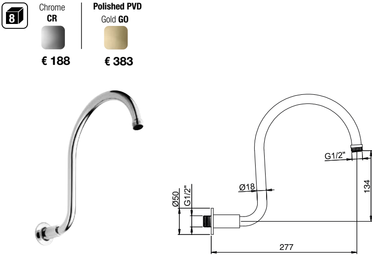
C021005 RETRO' - OTTONE RETRO' - BRASS
