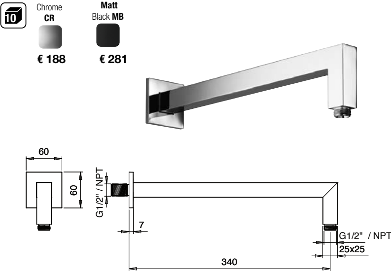
E021003 BRACCIO QUADRO CON ROSONE QUADRO L340 - OTTONE SQUARE ARM WITH SQUARE ROSETTE L340 - BRASS
