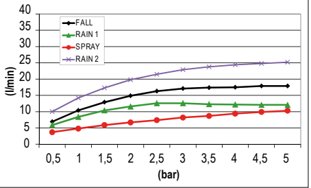
diagramma di portata | flowrate
