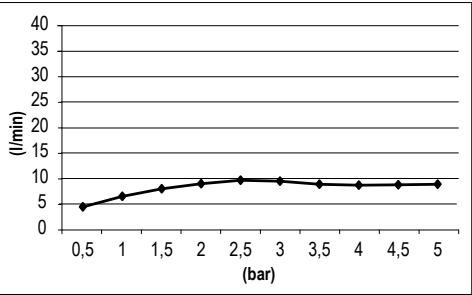
diagramma di portata | flowrate
