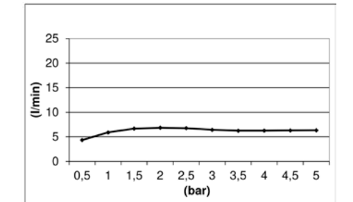
diagramma di portata | flowrate
