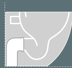
ACA033 CURVA TECNICA A 90° REGOLABILE DA 7 A 14 CM ADJUSTABLE 90° ELBOW FROM 7 TO 14 CM
