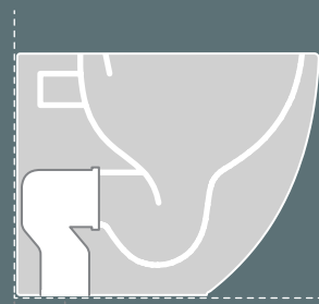
ACA005 CURVA TECNICA S SCARICO FISSO 15 CM ELBOW AT FLOOR S FIXED DRAIN 15 CM
