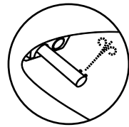
igiene posteriore posterior cleansing
