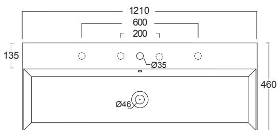
NEW 343370101 Lavabo SPY 121x45 NEW 343370101 Washbasin SPY 121x46
