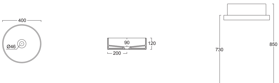
31140101 Lavabo HIDE Circle 31140101 Washbasin HIDE Circle
