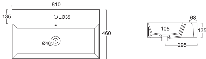
34330101 Lavabo SPY 81x46 34330101 Washbasin SPY 81x46
