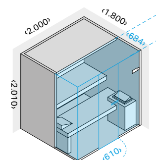
ДВЕРЬ ВПРАВО
