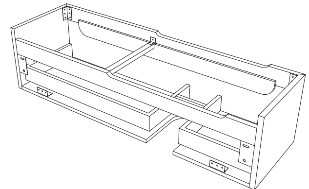
ASSONOMETRIA VISTA POSTERIORE
