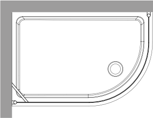
Cabina doccia semicircolare DX per piatto doccia 80x120 DX. Shower enclosure for corner shower-tray 80x120 right side.
