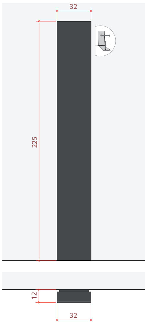
Vista laterale: Side view: Vue latérale: Seitenansicht: Vista lateral:
