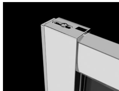
Premium Pro – стандартный U-образный профиль со стороны стационарной стенки.
