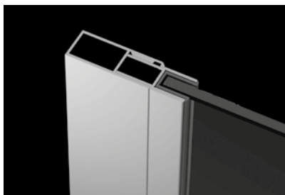
Carena – профиль +2 см. Стандартный U-образный профиль заменяется расширительным профилем P01-133195001.
