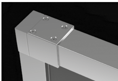
Idea 6 – профиль +2 см. Стандартный профиль заменяется расширительным профилем P01-ID-001-01.
