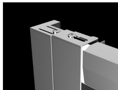
Premium Pro – профиль +2 см. Расширительный профиль добавляется к стандартному U-образному профилю со стороны двери P01-293199801.
