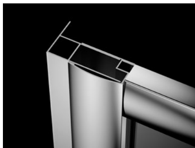
Premium Plus DWD – профиль + 2 см. Стандартный U-образный профиль заменяется расширительным профилем P01-130190001.
