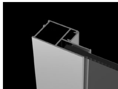
Torrenta, Eos – Профили + 2 см (кроме моделей Eos I, Torrenta PDJ). Стандартный U-профиль следует заменить на удлинительный профиль P01-284195001.
