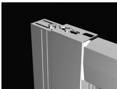
Premium Pro – профиль +2 см. Расширительный профиль добавляется к стандартному U-образному профилю со стороны стационарной стенки P01-293199801.
